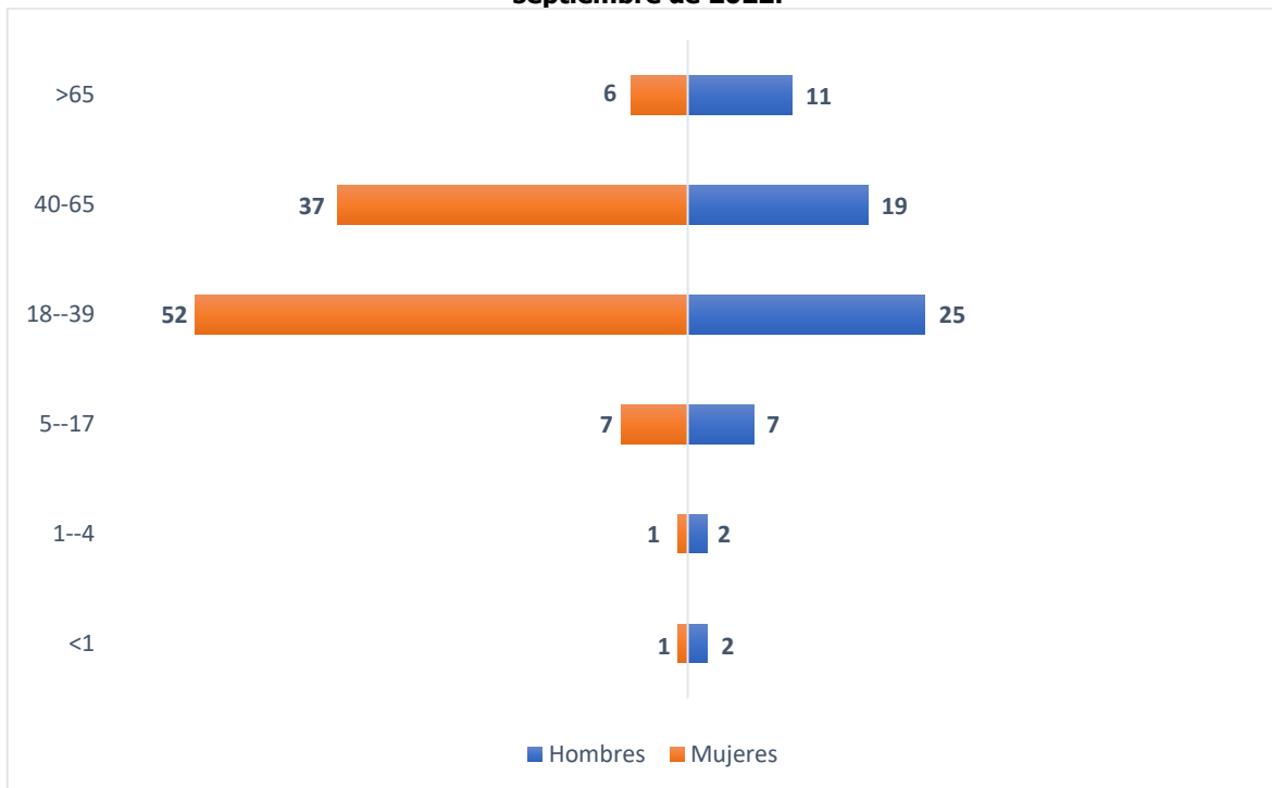
Gráfica 4. Casos de VOC de muestras secuenciadas localmente, del 15 de agosto al 04 de septiembre de 2022.
