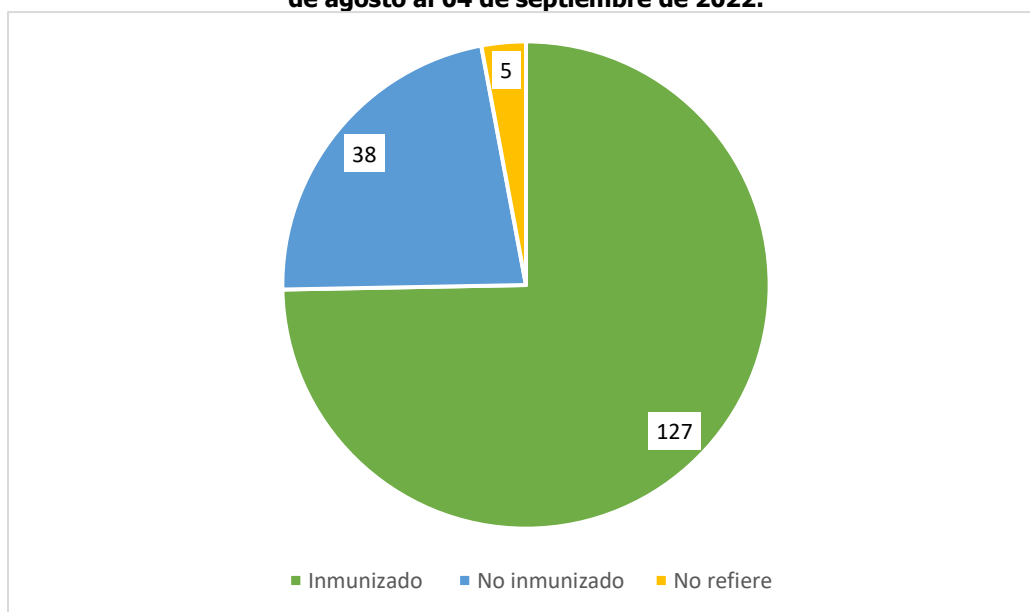
Gráfica 5. Porcentaje de casos inmunizados de VOC de muestras secuenciadas localmente, del 15 de agosto al 04 de septiembre de 2022.
