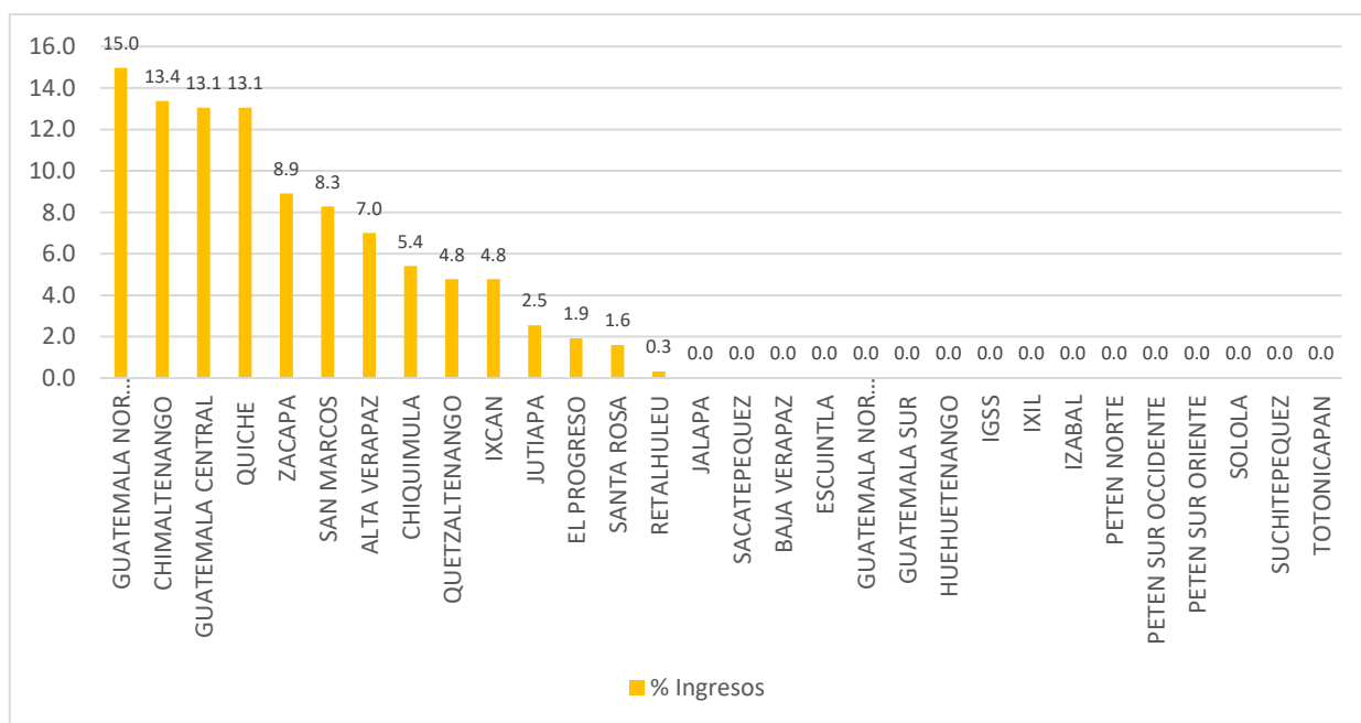
Gráfica 1. Porcentaje de muestras seleccionadas para el ingreso al LNS para el proceso de secuenciación, por área de salud, del 15 de agosto al 04 de septiembre de 2022
